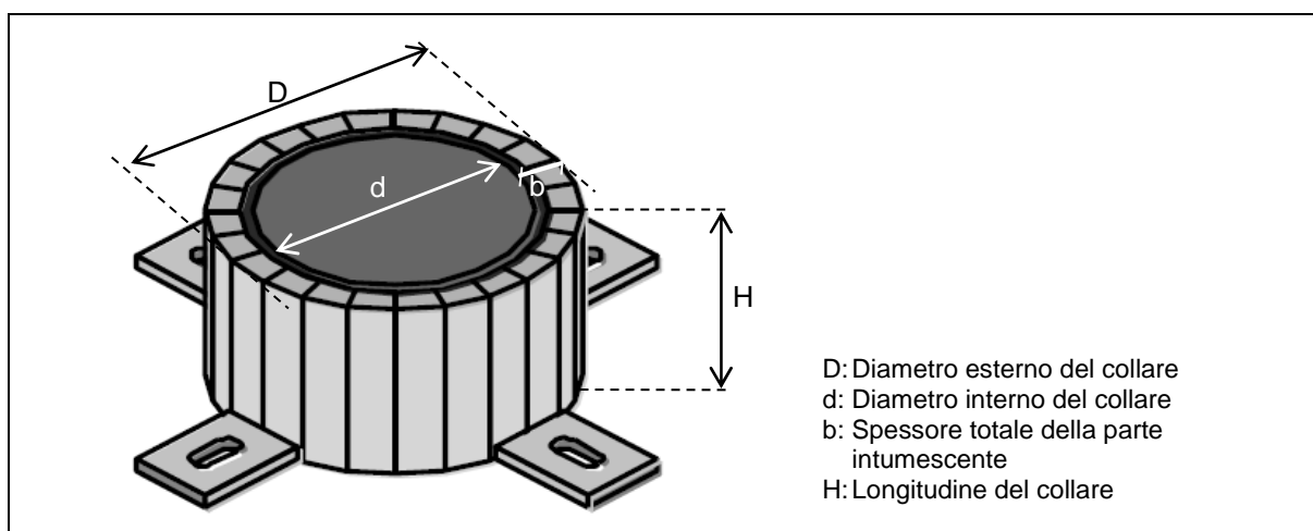
Figura A.1: Dimensioni dell'AF Collar.
