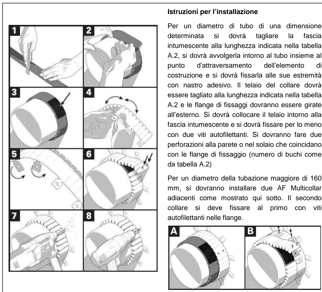
Figura A.3: Passaggi dell'installazione dell' AF Multicollar.
