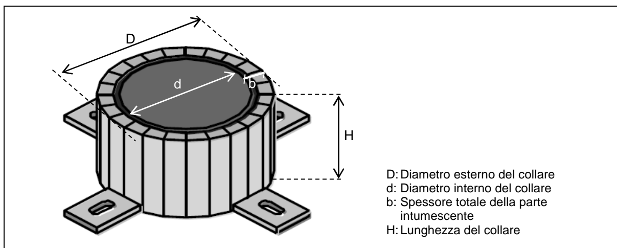
Figura A.2: Dimensioni dell'AF Multicollar (installato).
