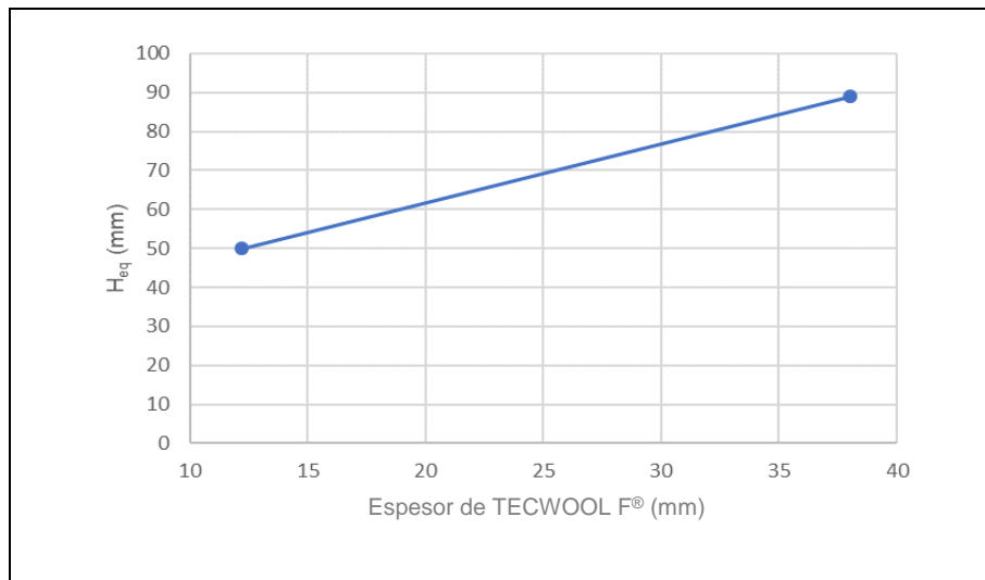
Figura A.2.3: Esesor equivalente de hormigón (90 minutos).
