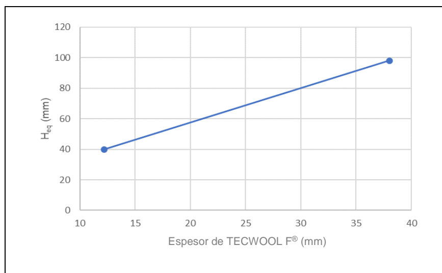
Figura A.2.5: Esesor equivalente de hormigón (180 minutos).
