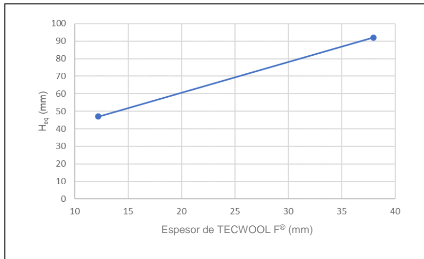
Figura A.2.4: Esesor equivalente de hormigón (120 minutos).
