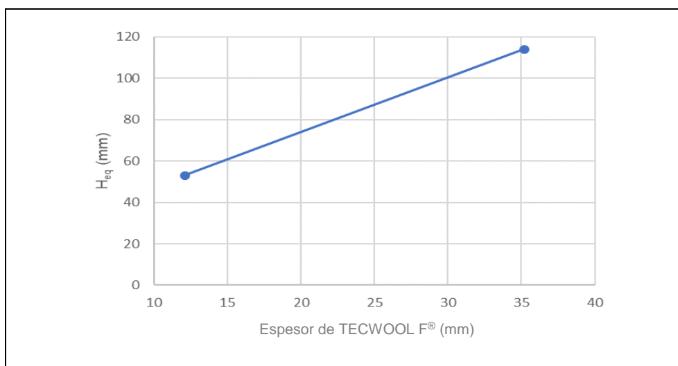
Figura A.2.8: Esesor equivalente de hormigón (90 minutos).
