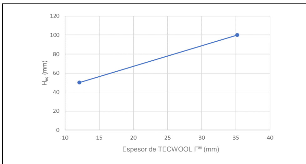
Figura A.2.7: Esesor equivalente de hormigón (60 minutos).
