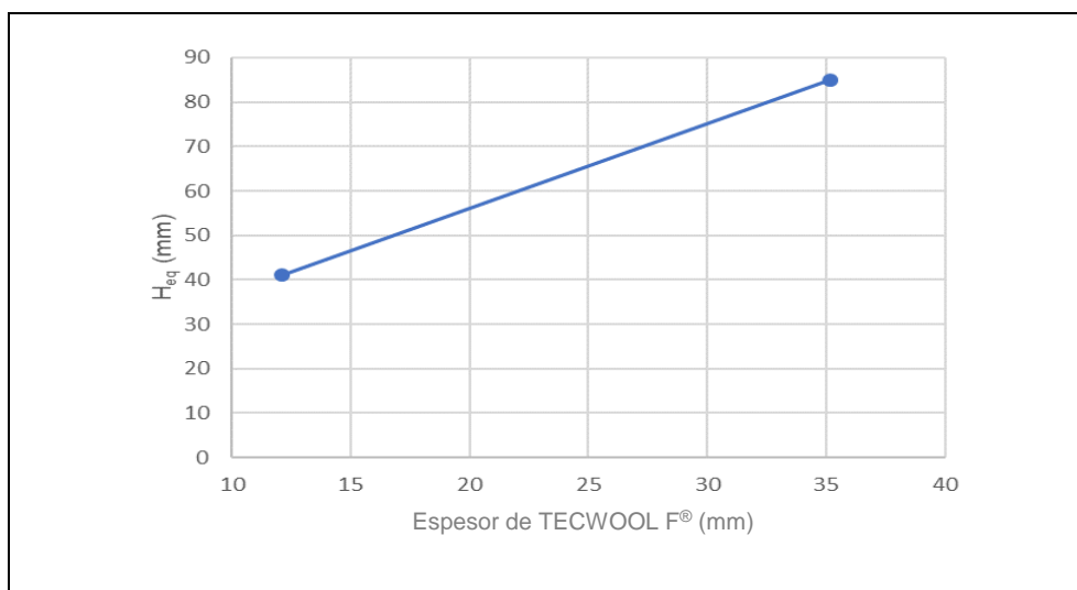
Figura A.2.6: Esesor equivalente de hormigón (30 minutos).
