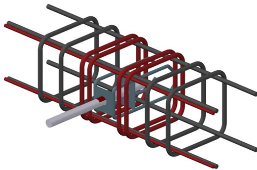
Figura 5.5: Disposición de los cercos de la armadura de suspensión y armadura de la viga de borde. Vista tridimensional.
