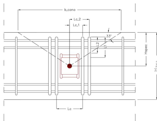
Figura 5.2: Modelo geométrico de disposición de armaduras de suspensión a ambos lados del vástago.
