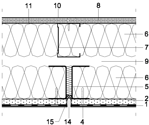
Figura 5.1.3: Junta de control superficial del sistema de doble hoja.
