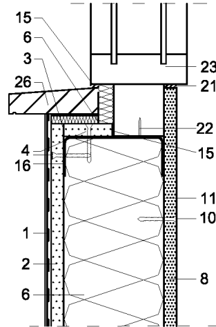
Figura 5.2.11: Alféizar del sistema de hoja simple.
