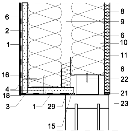
Figura 5.1.11: Dintel del sistema de doble hoja.
