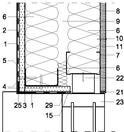
Figura 5.1.7: Jamba del sistema de doble hoja.
