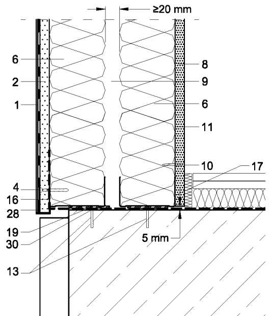
Figura 5.1.10: Arranque del sistema de doble hoja.
