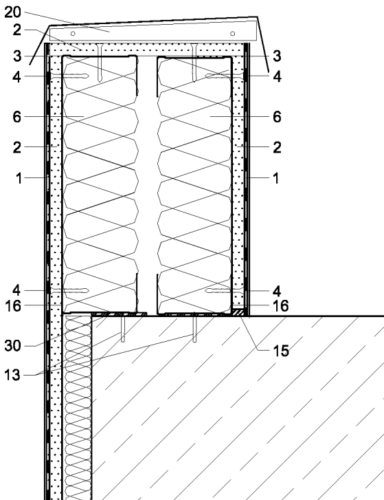
Figura 5.1.13: Coronación del sistema de doble hoja.
