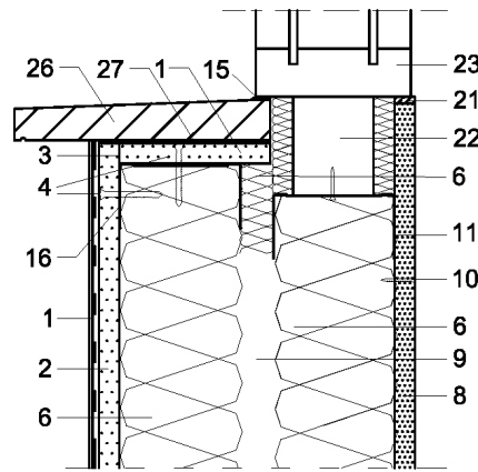
Figura 5.1.12: Alféizar del sistema de doble hoja.
