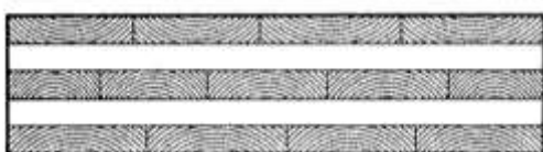
Figura A1.2: Estructura principal de un panel de madera maciza de 5 capas.
